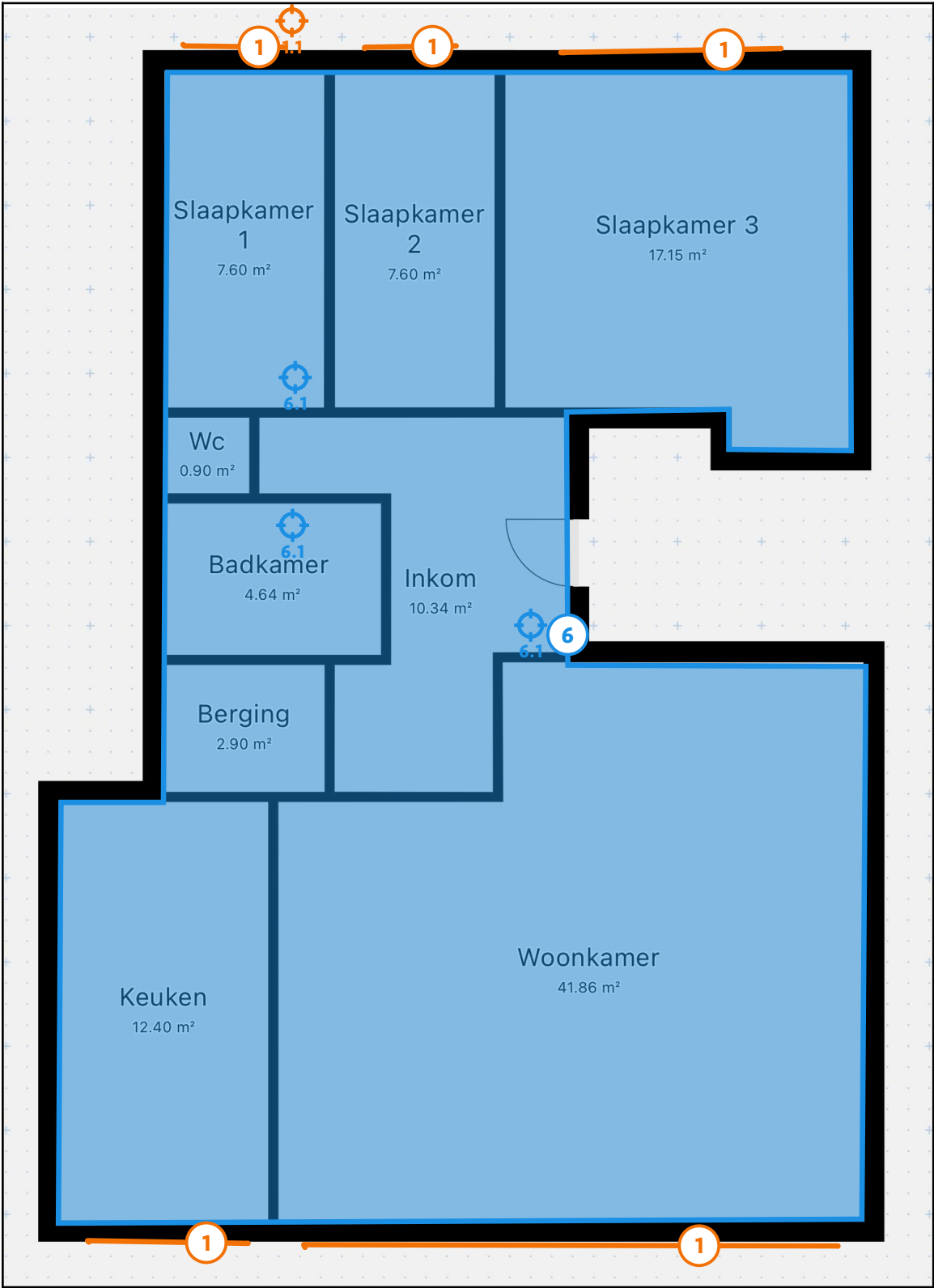
Legende van plan 2.3: Appartement pleisterwerk plafonds - mastiek
